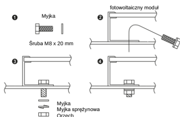
Fig. A3-1: Elementy do Śruba & Orzech
