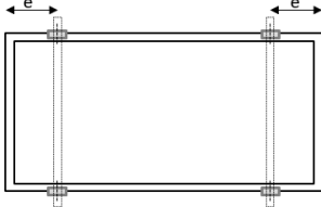
Fig. A2: Pozycja klemy przy mocowaniu na długim boku (4 klemy)
