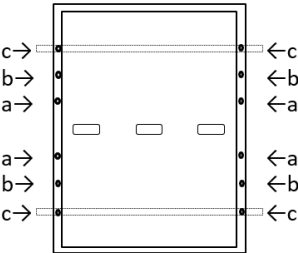
Fig. A3: Położenie otworów montażowych
