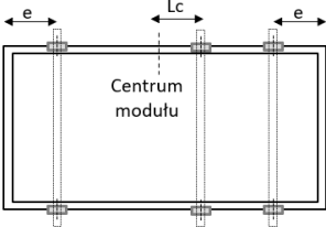
Fig. A1: Pozycja klemy przy mocowaniu na długim boku (6 klemy)
