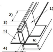
Rys. 4. Wymagania dotyczące klamer (zacisków)
