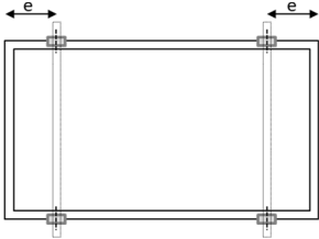
Rys. A2: Pozycja klemy przy mocowaniu na długim boku (4 klemy)
