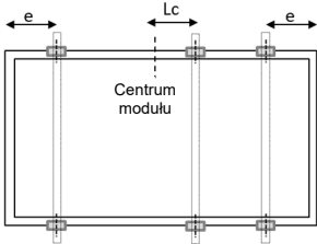
Rys. A1: Pozycja klemy przy mocowaniu na długim boku (6 klemy)
