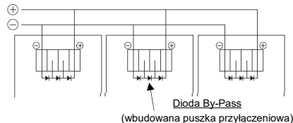
Rys. 2. Połączenie RÓWNOLEGLE daje większy prąd.
