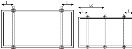
Fig. A1: Pozycja klemy przy mocowaniu na długim boku
