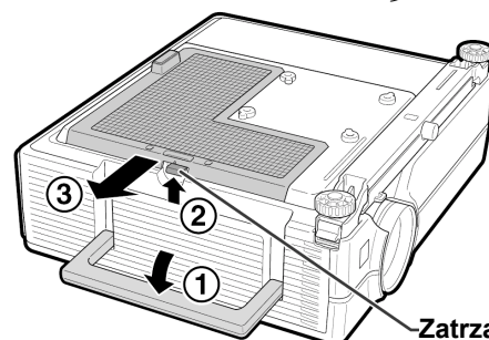
Zatrzask
