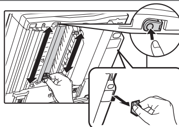
Rolka pobierająca papier
