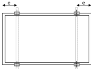
Rys. A1: Pozycja klemy przy mocowaniu na długim boku Szyny montażowe prostopadłe do dłuższej ramy
