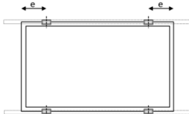
Rys. A2: Pozycja klemy przy mocowaniu na długim boku Szyny montażowe równoległe do dłuższej ramy
