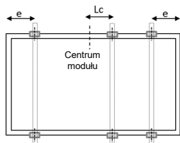
Rys. A1: Pozycja klemy przy mocowaniu na długim boku (6 klemy)
