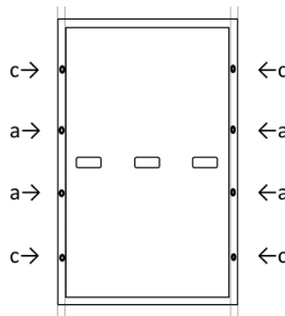
Rys. B2: Położenie otworów montażowych
