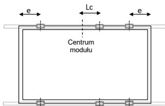
Rys. A2: Pozycja klemy przy mocowaniu na długim boku (6 klemy)
