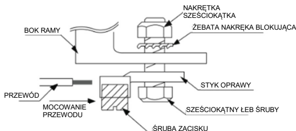
Rys. 3. Przykład dopuszczalnego uziemienia
