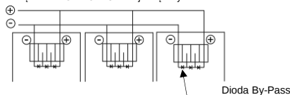
Rys. 2. Połączenie RÓWNOLEGŁE daje większy
