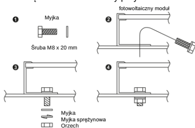
Fig. A3-1: Elementy do Śruba & Orzech
