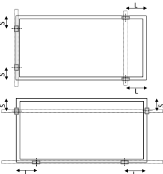
Fig. B: Pozycja klem przy mocowaniu na krótszym i dłuższym boku
