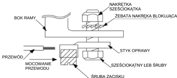
Rys. 3. Przykład dopuszczalnego uziemienia
