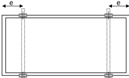
Fig. A1: Pozycja klem przy mocowaniu na długim boku
