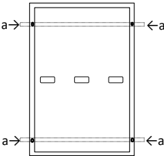
Fig. A3: Położenie otworów montażowych
