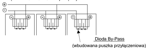
Rys. 2. Połączenie RÓWNOLEGLE daje większy
