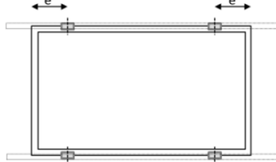
Rys. A2: Pozycja klem przy mocowaniu na długim boku Szyny montażowe równoległe do dłuższej ramy
